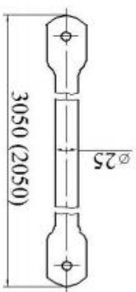
Горизонтальная связь (3)
