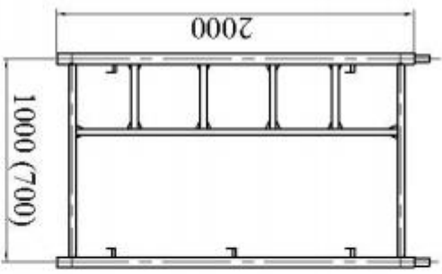
Рама с лестницей (2)
