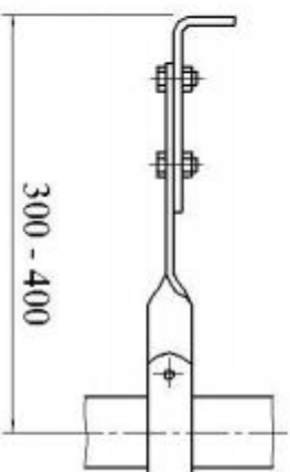
Кронштейн крепления (6)
