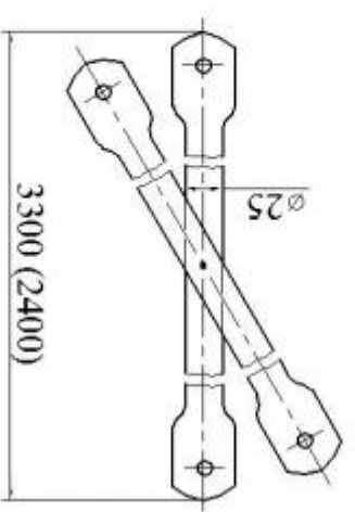
Диагональная связь (4)
